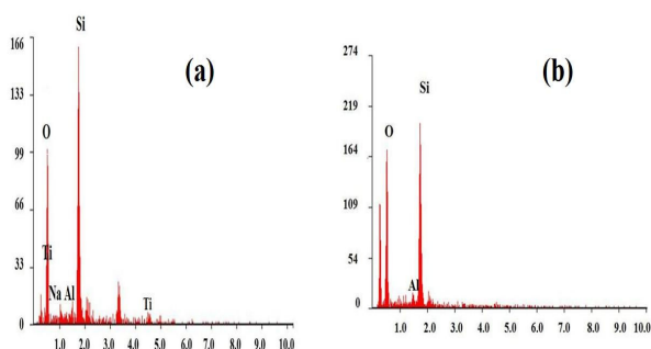
Fig. 6 EDAX results for (a) 15 % TiO_2 -NaY and, (b) Ti_4 -NaY
