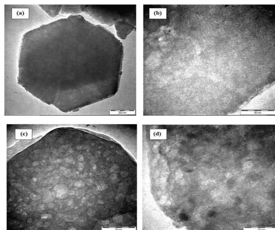
Fig. 7 TEM images for (a and b) NaY, (c) 15 % TiO_2 -NaY and, (d) Ti_4 -NaY
