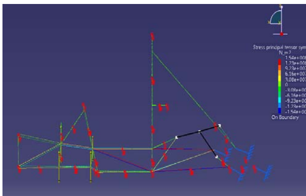
Fig. 18 Schneller frame (CATIA)
