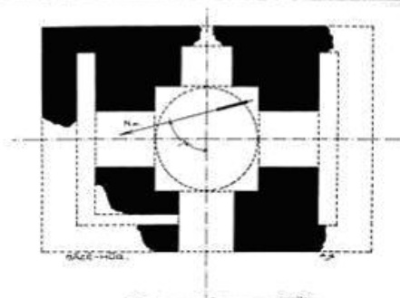
FIG. 29. PLAN DE L'ÉDIFICE DE BAZE-HÜR
