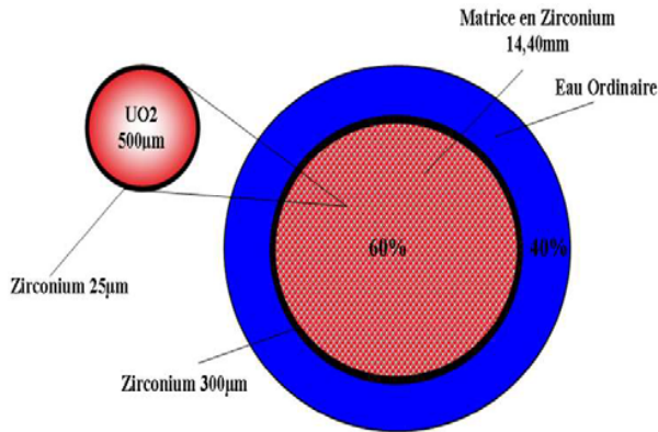
Fig 1 Cermet MFE parameters
