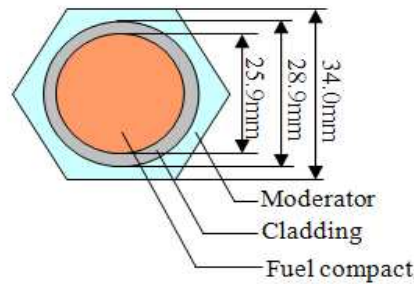
Fig. 2 Cermet MFE and cell parameters
