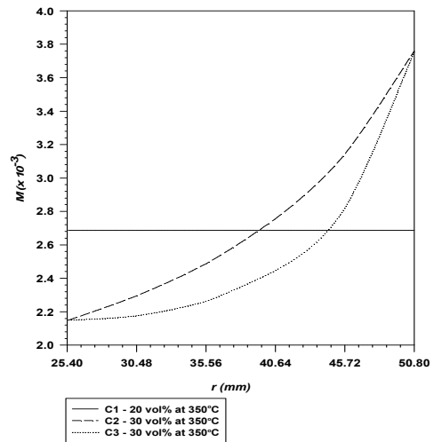
Fig. 3 Distribution of Creep Parameters M(r)
