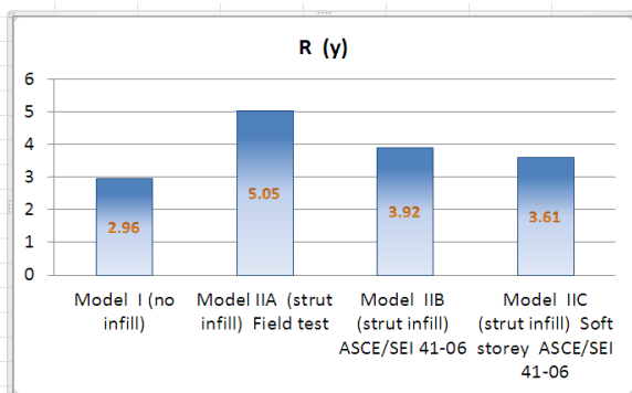
Fig. 18 (b) Y - Direction
