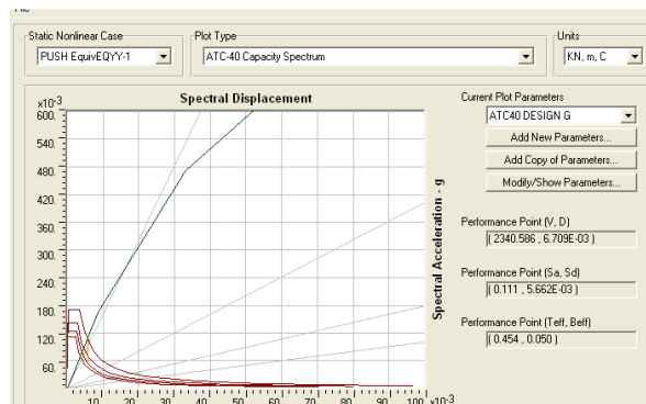
Fig. 17 (d) Model IIC (strut infill-Soft storey-ASCE/SEI 41), R=3.61
