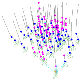
Fig. 13 (d) Model IIC (strut infill-Soft storey-ASCE/SEI 41)
