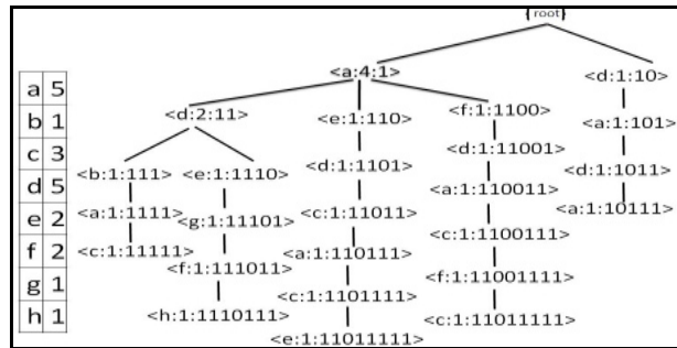
Fig. 1 RePLNI-tree
