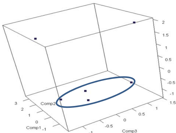
PCA
