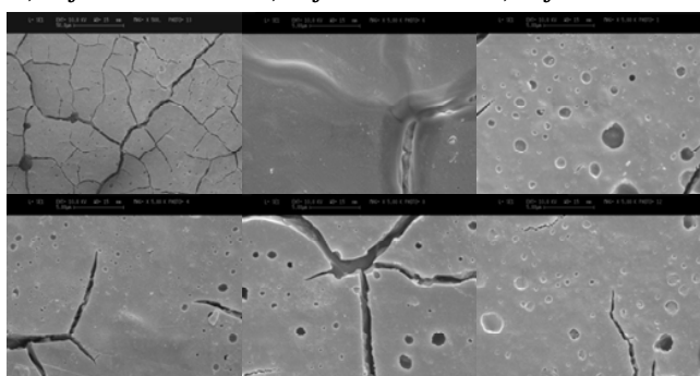
d) Fuji IX 168 h water e) Fuji IX 168 h P.J. f) Fuji IX 168 h wax
