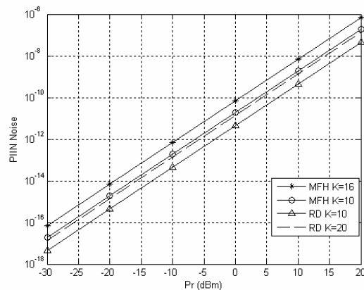
Fig. 4 PIIN versus P_r for versus OCDMA codes
