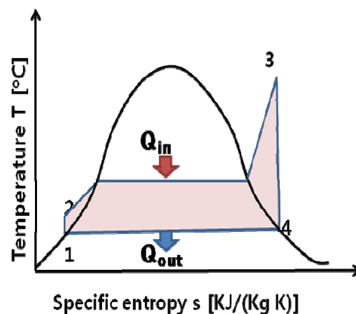
Fig. 2 T-s diagram
