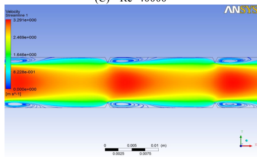
(D) Re=50000
