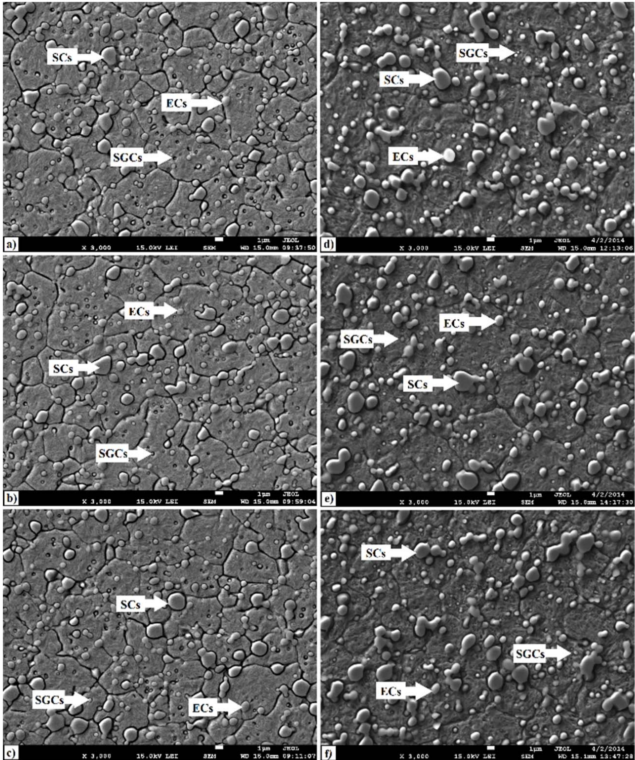
Fig. 2 SEM micrographs showing microstructure of Vanadis 6 ledeburitic steel (a) SIZT -140 °C/10 h, (b) SIZT -140 °C/24 h, (c) SIZT -140 °C/48 h, (d) SIZT -196 °C/10 h, (e) SIZT -196 °C/24 h, (f) SIZT -196 °C/48 h
