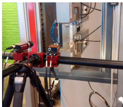
Fig. 3 Test setup
