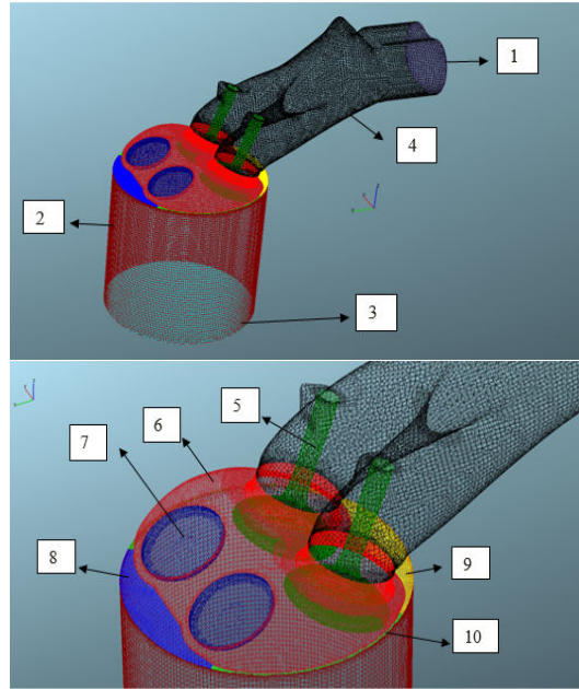
Fig. 1 Volume mesh
