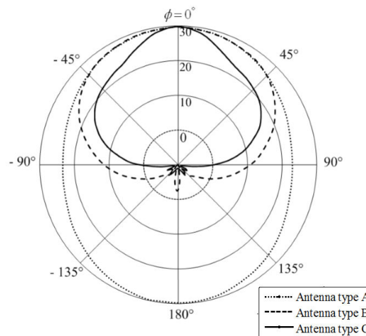
(b) H-Plane
