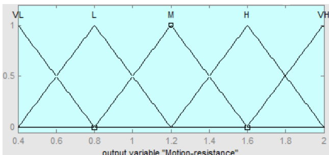
(d)motion resistance
