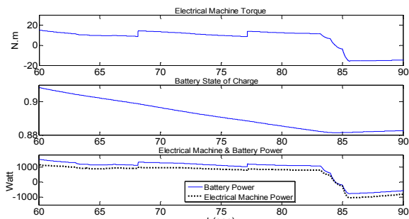
Fig. 18.b Fig. 18.a for 60^{sec} < t < 90^{sec}
