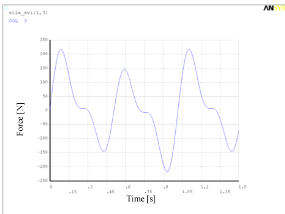
Fig. 20 Longitudinal force time record
