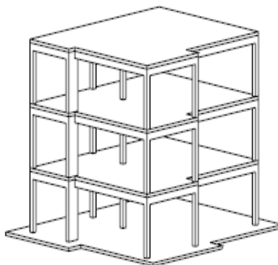
Fig. 4 The SPEAR frame, Actual Structure.
