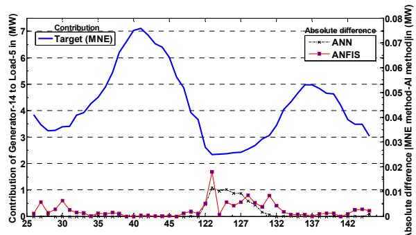
(d) Contribution to load at Bus 5
