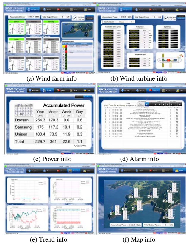
Fig. 9. CMS-Server software.
