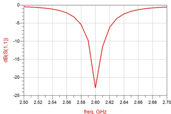
Fig. 4 Parameter S11 for 2.6 GHz
