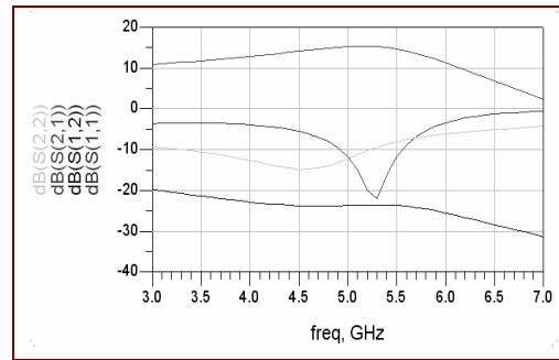
Fig. 9 S-Parameter Plot
