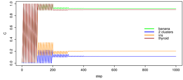
(a) Tuning of SVDD parameter C .
