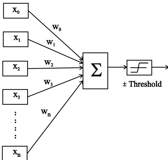
Fig. 2 Perceptron
