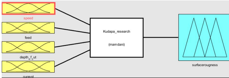
Fig. 3 Mamdani FIS
