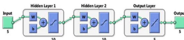
Fig. 3 ANN topology
