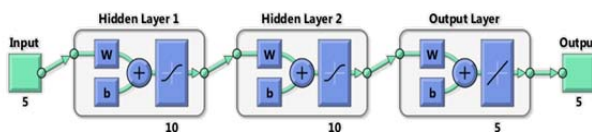
Fig. 3 ANN topology
