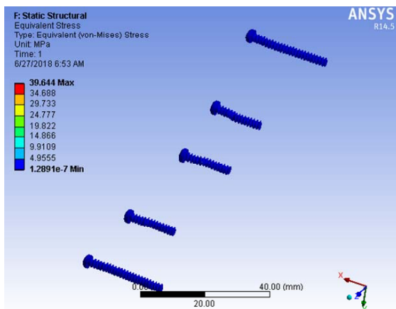
Fig. 5 (d) Von-Mises stress distribution in all screws
