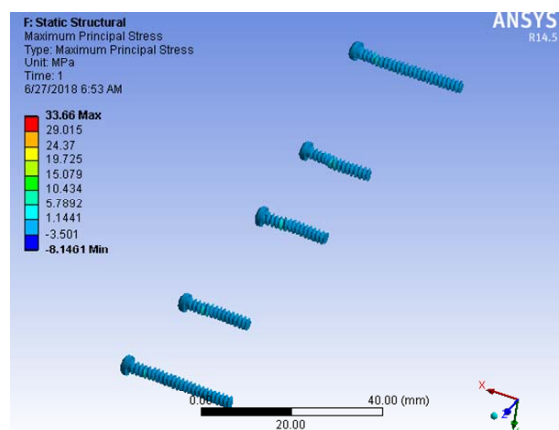
Fig. 6 (d) Maximum principal stress in all screws
