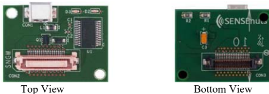
Fig. 4 Gateway module
