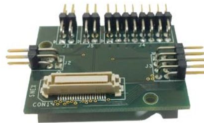
Fig. 7 Extender
