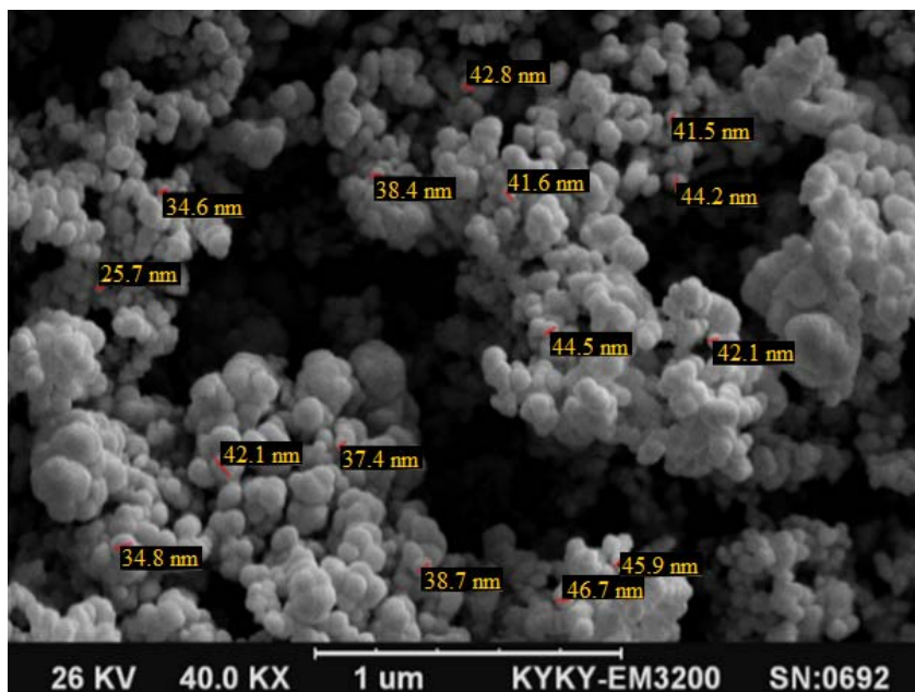
Fig. 3 SEM images of A-MNPs
