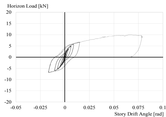
(d) H-SF specimen
