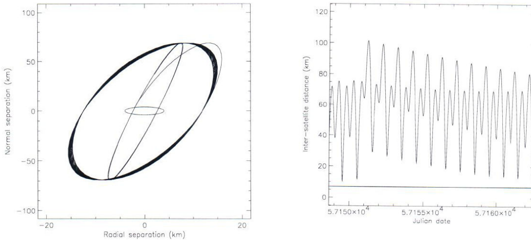
Fig. 15 (d) Scenario 4 – Change e_x and e_y and date of correction
