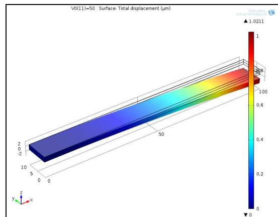
Fig. 6 Piezoelectric actuator
