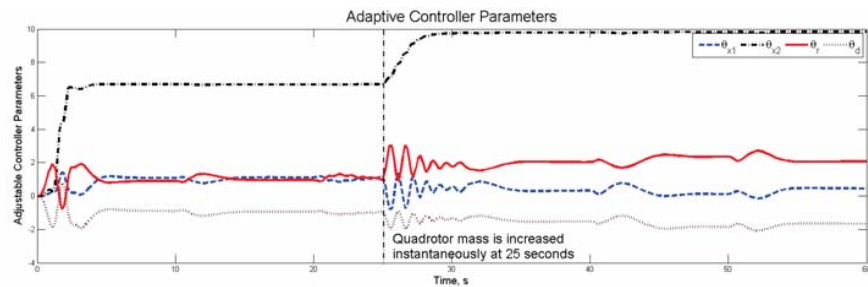
Fig. 5. MRAC Controller Parameters
