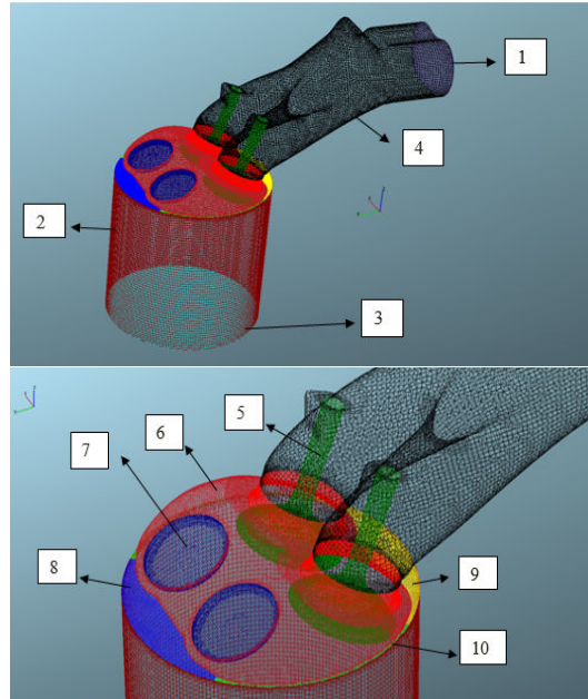
Fig. 1 Volume mesh
