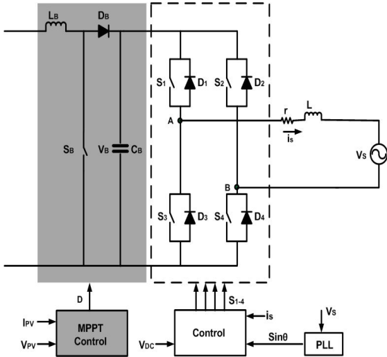
Fig. 1 SPI
