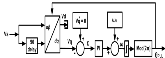
Fig. 3 PLL
