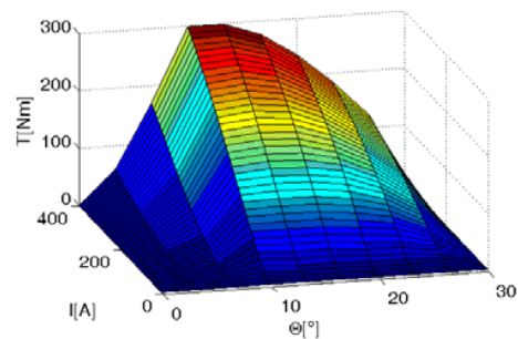
Fig. 3 Motor torque map
