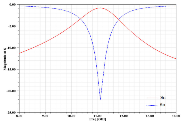
Fig. 4 Magnitude of S Parameters of ETDS
