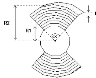
Fig. 9 Specifications rotor R 1 = 3 cm, R 2 = 5.7 cm, L = 2.4 cm, \alpha = 90°
