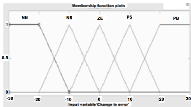
Fig. 4 Membership functions of parameter Vn.
