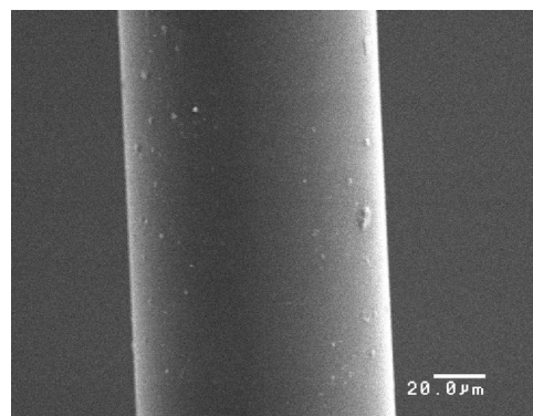
PA6-500 m/min
