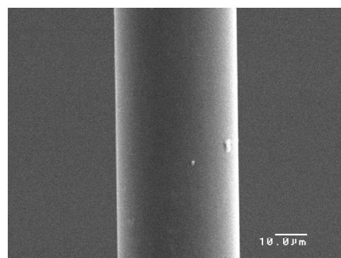
PA6-5000 m/min
