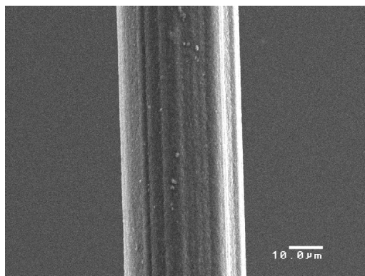
BiCo- 5000 m/min
