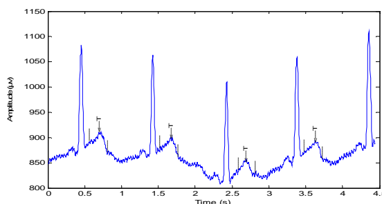
Fig. 5 Baseline drift (121.dat)
