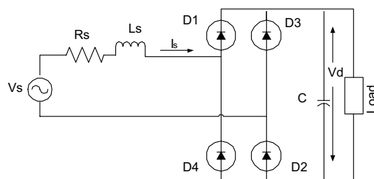
Fig. 1 Diode bridge rectifier circuit
