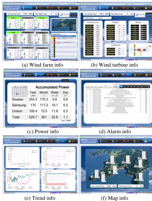
Fig. 9. CMS-Server software.
