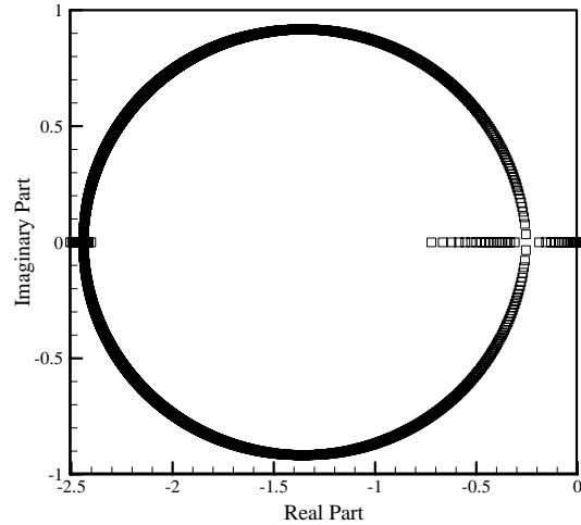
Fig. 6 The Eigenvalues in \lambda -plane
