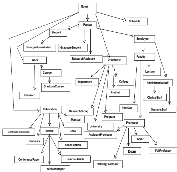
Fig. 4 Univ-Bench Ontology
