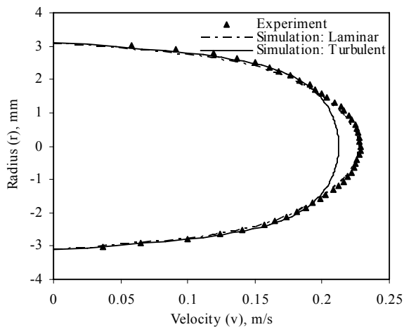
a. Re = 155
