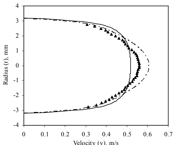
c. Re = 390
