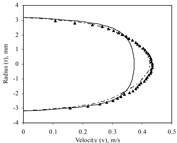
b. Re = 270
