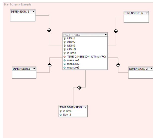
Fig. 1 Star Schema
