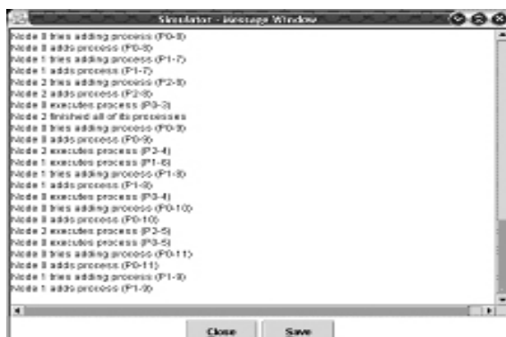
Fig. 7 Message Window
